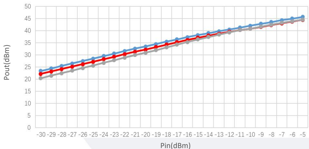
Pout@Pin
